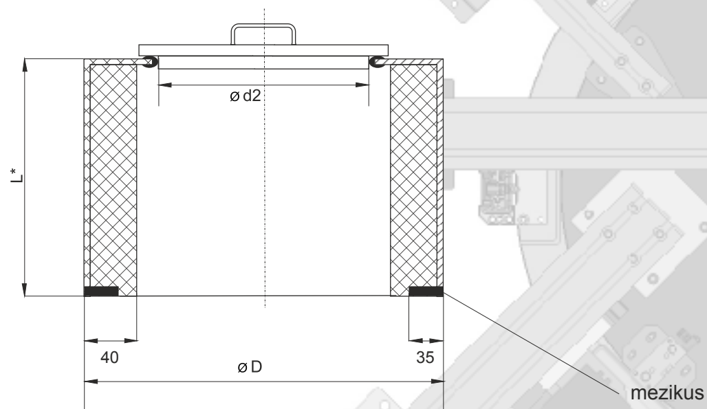
Rozměrový náčrtek
